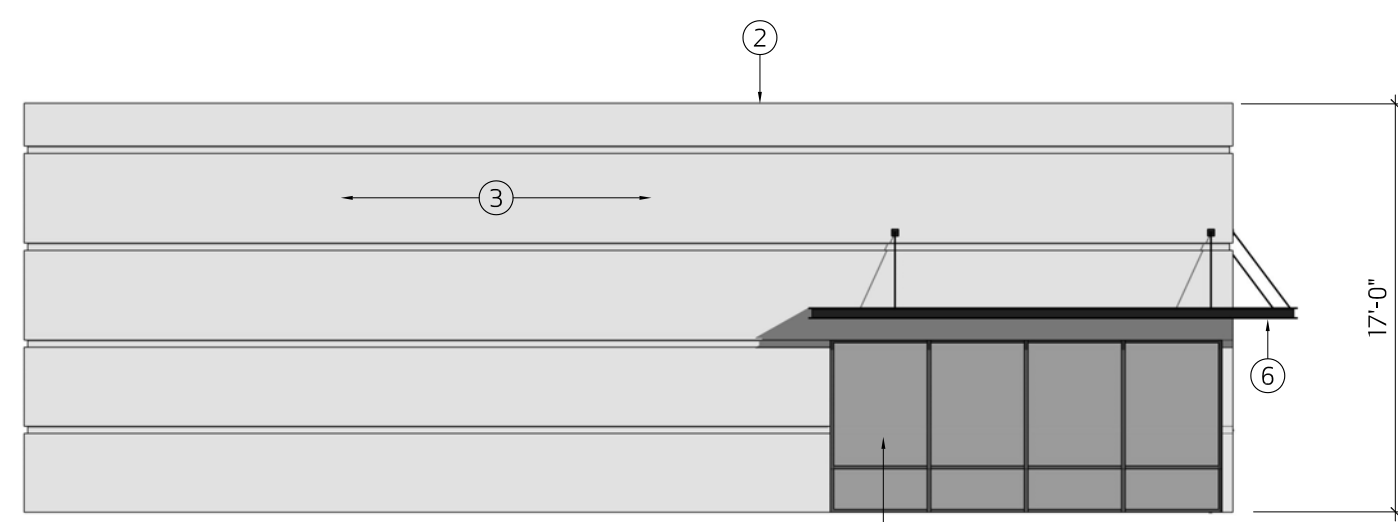
1 WEST ELEVATION SCALE: 1/8"=1'-0"
